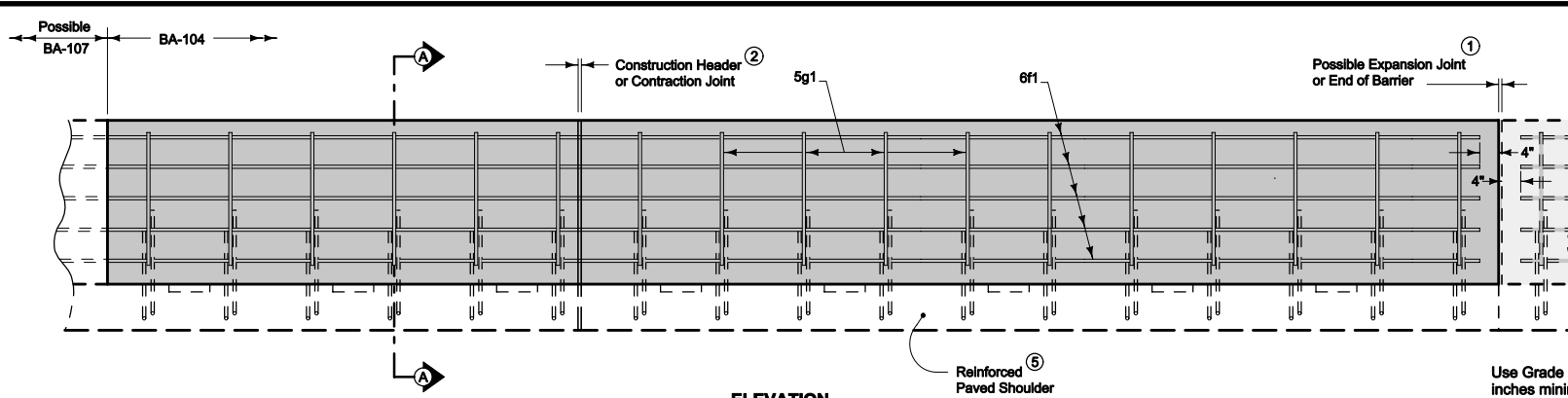
ELEVATION
