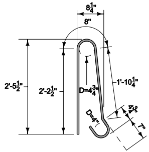
5g1 BENT BAR
